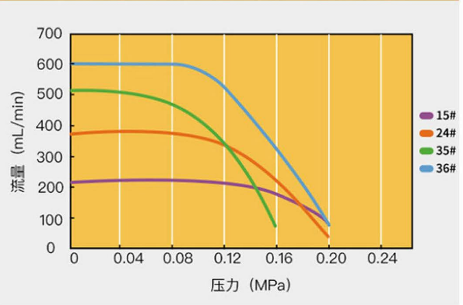
DZ25-3L泵头压力/流量曲线图 (100rpm)
